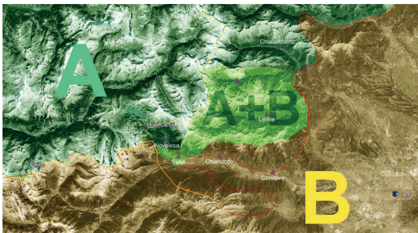
Figure 5 : Frêne : distribution des types * frèno (A) et frâisse (B) dans l'aire de contact entre francoprovençal et occitan-piémontais (val de Susse, vallées de Lanzo).
