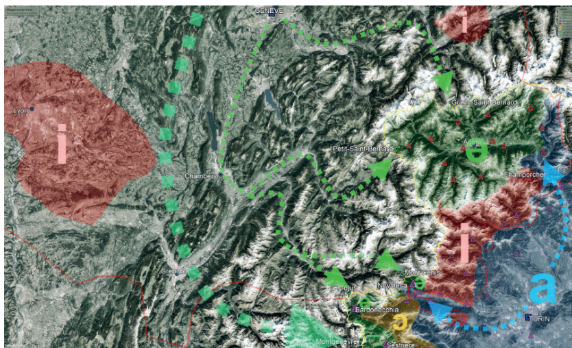
Figure 9 : Feuille : issues de /a/ atone final (<folia) dans le secteur francoprovençal ; cols alpins et lignes de pénétration des issues gallo-romanes septentrionales (en vert) et italo-romanes (en bleu).
