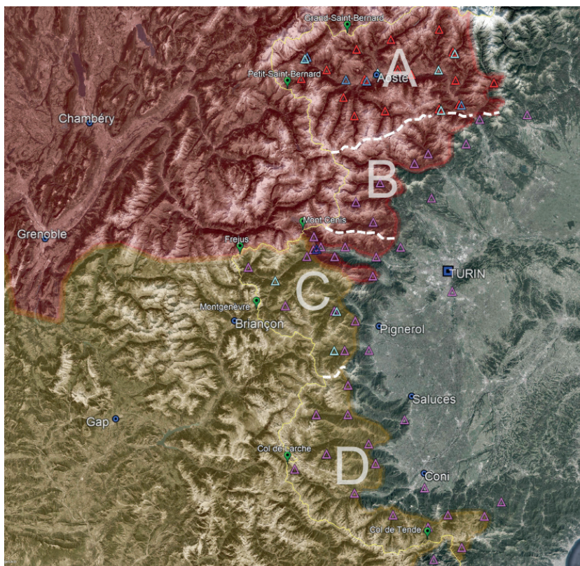
Figure 1 : L'aire gallo-romane « italienne », son appartenance linguistique (rouge : francoprovençal ; jaune : occitan), ses zones géographique (A, B, C, D : voir texte) et sa couverture géolinguistique (triangles en nuance bleu : atlas français – ALF, ALJA, ALMURA – ; triangles rouges : APV ; triangles violets : ALEPO).
