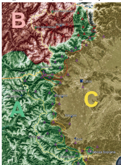
Figure 7 : Donner : l'aire gallo-romane « italienne » et la distribution des types étymologiques donare (A), baiulare (B) et dare (C) ; en bas, mise en évidence, l'aire des parlers du kje (Frabosa Soprana).
