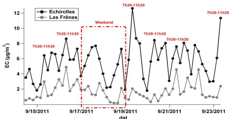
Figure 1 : Évolution temporelle du carbone élémentaire (EC) à Grenoble. Temporal evolution of elemental carbon (EC) in Grenoble.
