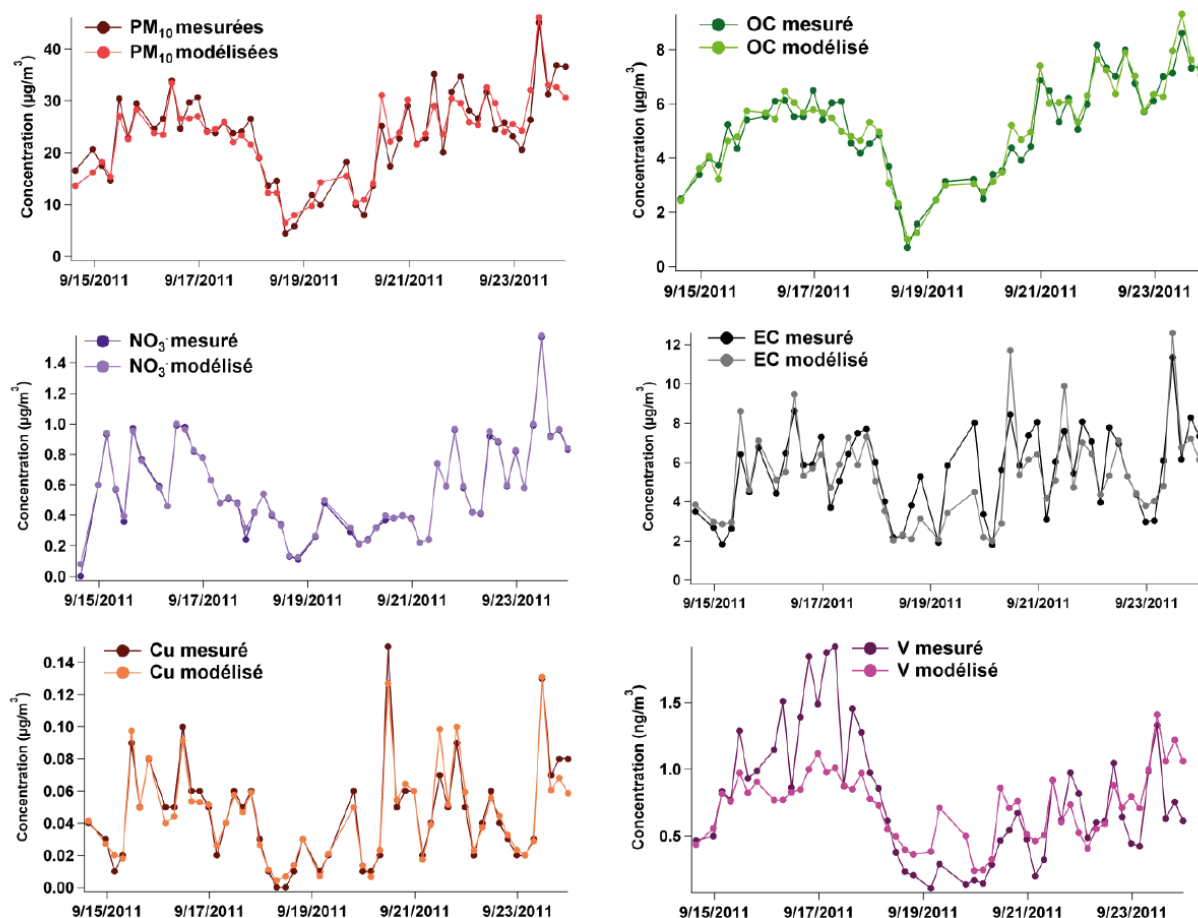
Figure 2. Concentrations mesurées et reconstruites avec la solution retenue pour le modèle PMF, pour quelques espèces importantes des PM10.
